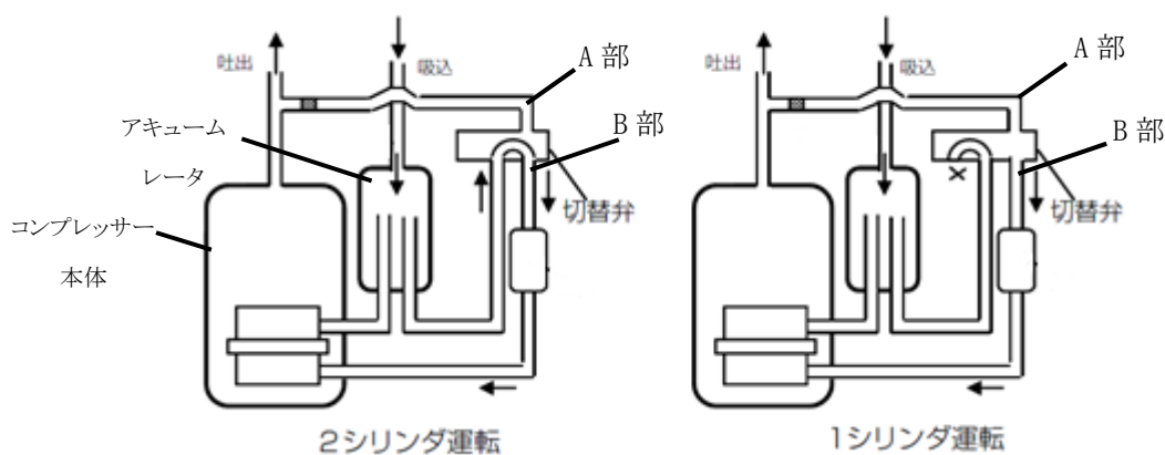
図 C.1 2 シリンダ運転と 1 シリンダ運転
