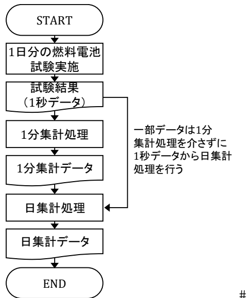
図1 燃料電池試験データの集計処理フロー
