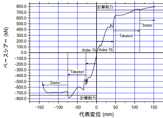
図 3 包絡線(基礎固定時)
