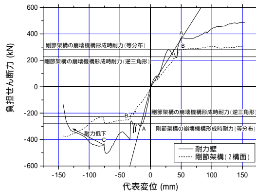
図 7 負担水平力(基礎固定時)
