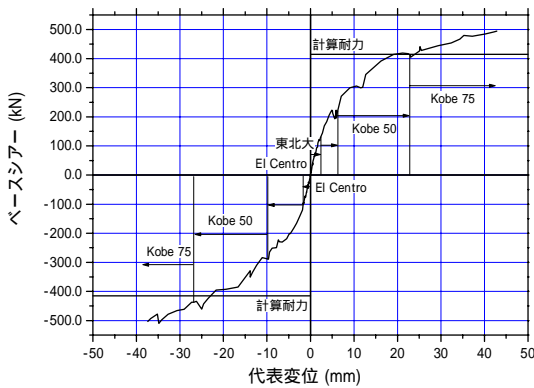
図 2 包絡線(基礎回転時)
