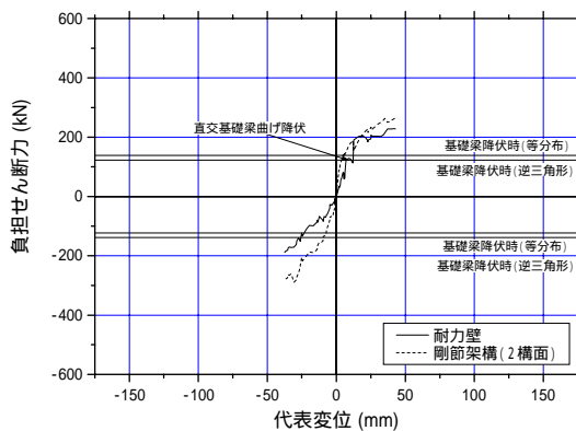
図 6 負担水平力(基礎回転時)
