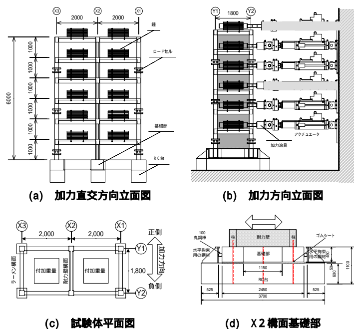
図 1 試験体形状・加力概要
