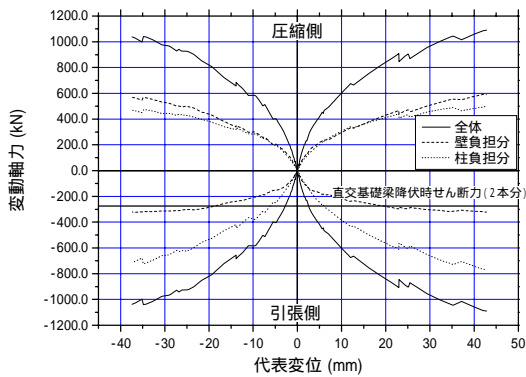
図 4 負担変動軸力(基礎回転時)
