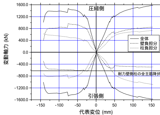
図 5 負担変動軸力(基礎固定時)
