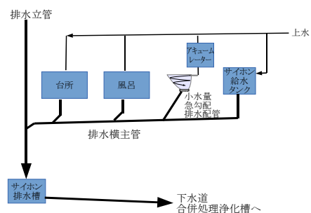
図1 下水道に対応した超節水型衛生設備システム (構成例)
