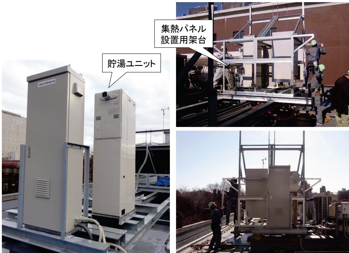
図 7.5.1.4 試験対象機の屋上試験装置への設置（架台準備）
