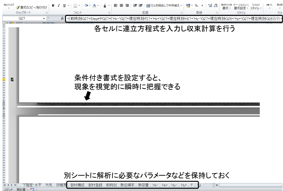
図 7.3.3.1 Excelによる2次元熱伝導解析の例
