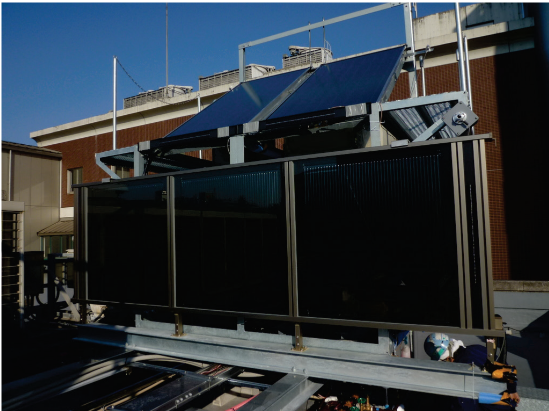
図 7.5.1.7 試験対象機の屋上試験装置への設置 (完了状態)
