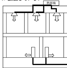
<セントラル(全館)空調システム> 1つの熱源機で複数の箇所の冷暖房を行う。
