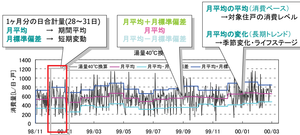
図 7.4.2.7 実住宅における給湯消費の変動
