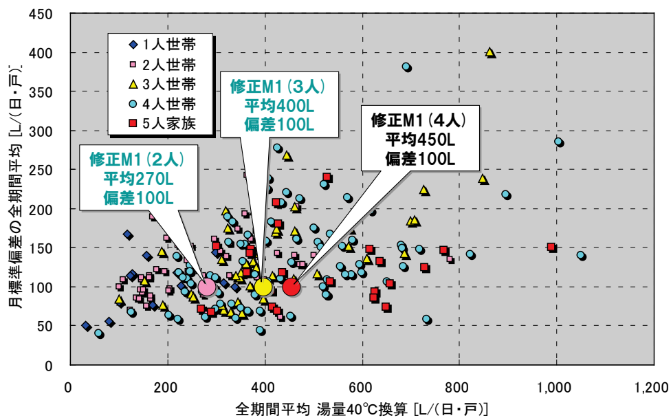
図 7.4.2.8 実測住戸における湯消費の平均（横軸）と日変動（縦軸）
