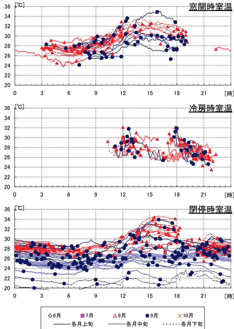
図 7.1.5.1 【住戸①】 各モードでの室温の推移 (8/12~9/24)
