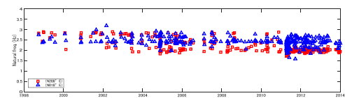
図 5.2 固有振動数 (6F/GL) の経年推移
