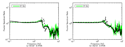
図 6.9 311 地震と震度 2 の地震の比較(1F/G) ※実線: 本震後、破線: 本震前
