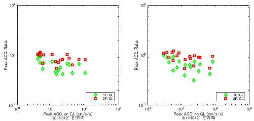
図 3.4 GL の最大加速度と 1F/QL 及び 3F/QL の最大加速度比の関係
