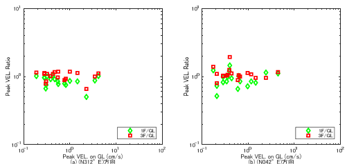
図 3.5 GL の最大速度と 1F/QL 及び 3F/QL の最大速度比の関係
