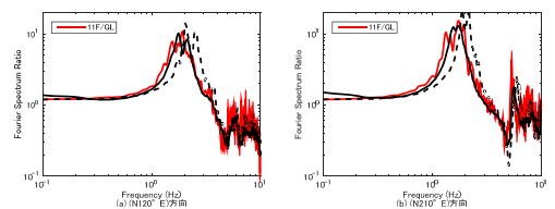
図 6.7 311 地震と震度 2 の地震の比較(1F/G) ※実線: 本震後、破線: 本震前
