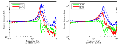
図 6.9 震度2の記録の平均スペクトル比(311前後) ※実線: 本震後、破線: 本震前
