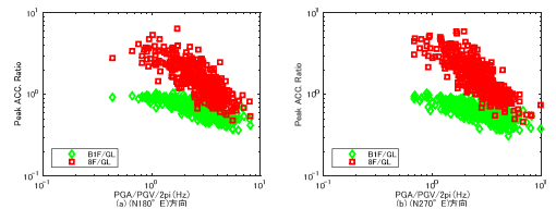
図 4.1 等価卓越振動数 (FA) と最大加速度比 (8F/GL, BIF/GL) の関係
