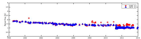
図 5.1 固有振動数 (8F/BIF) の経年推移
