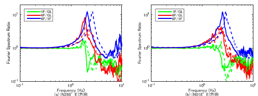
図 6.11 震度4の記録の平均スペクトル比(311前後) ※実線: 本震後、破線: 本震前
