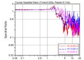
図 7.5 1階 (O1F) の地表 (GL) に対するフーリエ振幅スペクトル比
