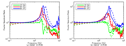
図 6.10 震度3の記録の平均スペクトル比(311前後) ※実線: 本震後、破線: 本震前
