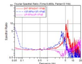
図 7.7 5階(O5F)の1階(O1F)に対するフーリエ振幅スペクトル比
