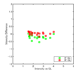
図 3.6 GL の最大震度と 1F/QL 及び 3F/QL の計測震度差の関係
