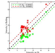
図 3.3 GLの計測震度と1F及び11Fの計測震度の関係
