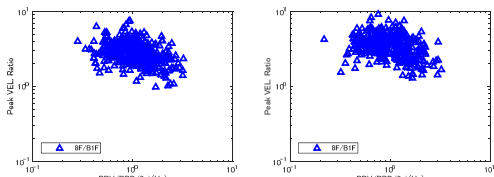
図 4.4 等価卓越振動数 (FV) と最大速度比 (8F/BIF) の関係
