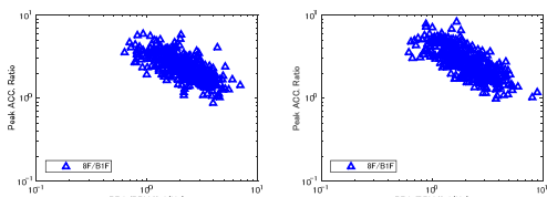
図 4.3 等価卓越振動数 (FA) と最大加速度比 (8F/BIF) の関係
