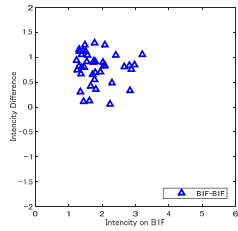
図 3.12 BIF の計測震度と 3F-BIF の計測震度差の関係
