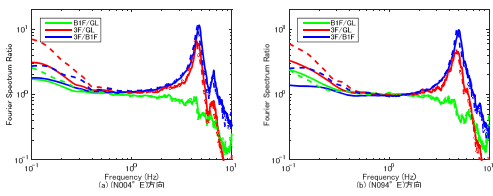
図 6.1 震度毎の平均フーリエスペクトル比(311 後) ※実線: 震度 2, 破線: 震度 3
