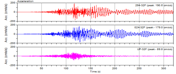
図 7.3 32階 (B2F) の加速度記録
