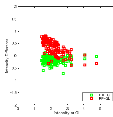
図 3.6 GL の最大震度と BIF/GL 及び RF/GL の計測震度差の関係
