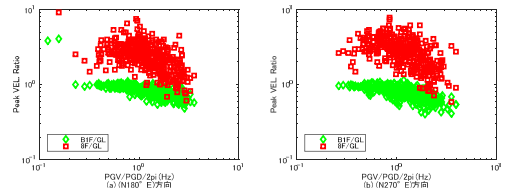
図 4.2 等価卓越振動数 (FV) と最大速度比 (8F/GL, BIF/GL) の関係
