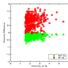
図 3.6 GL の最大震度と BIF/GL 及び 8F/GL の計測震度差の関係
