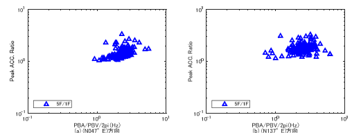
図 4.3 等価卓越振動数 (fa) と最大加速度比 (SF/1F) の関係
