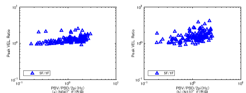
図 4.4 等価卓越振動数 (fv) と最大速度比 (SF/1F) の関係
