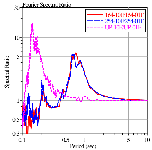
図 4.2-18 10階(10F)の1階(01F)に対するフーリエスペクトル比
