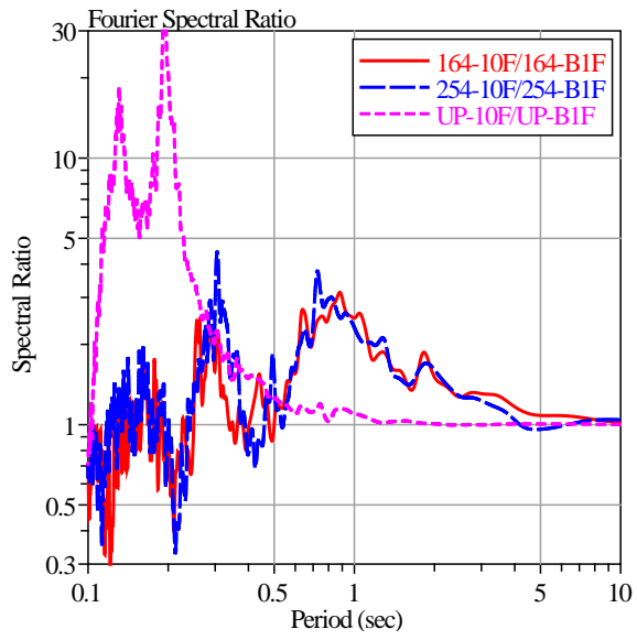
図 4. 2-19 10 階 (10F) の基礎 (B1F) に対するフーリエスペクトル比
