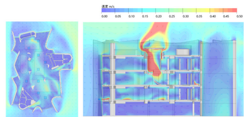
自然換気の経路を把握→採風に最も有効な窓の位置を決定
