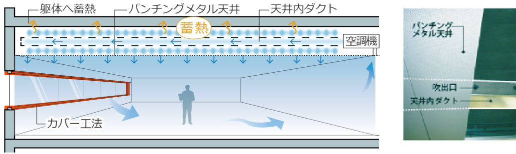
オフィス空調の天井内チャンパーによる多孔吹出し天井の概念図
