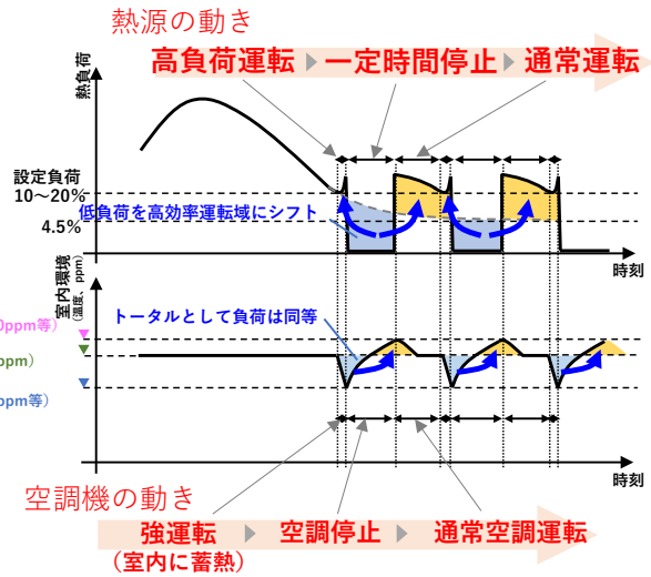
低負荷時高効率熱源制御システム概念図
