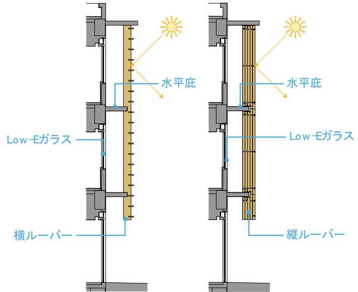
ルーバー断面 (左：南面、右：その他方位)
