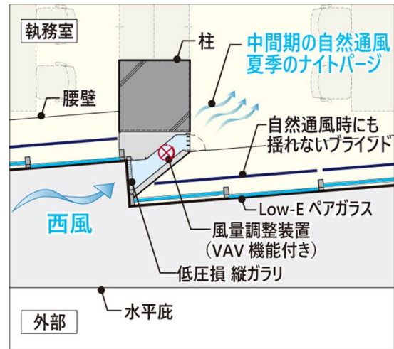
自然通風取入口の平面ディテール
